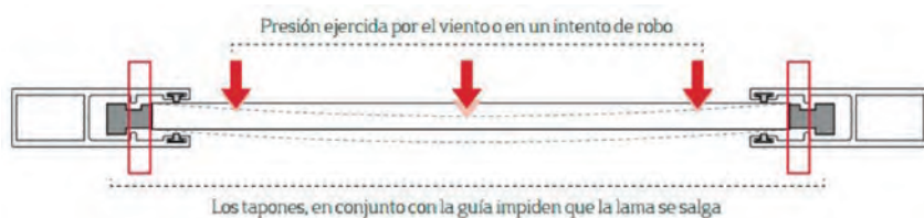
Figura 76. Sección horizontal de una lama y guías en sistema de alta seguridad, mostrando los tapones empotrados en la guía.
