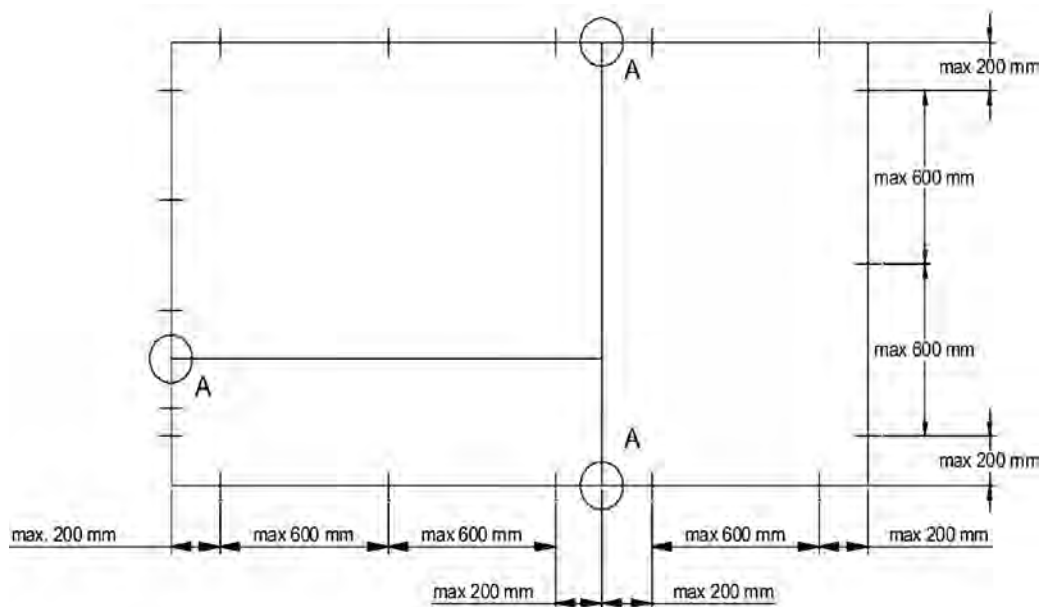
Figura 7. Posicionamiento de las fijaciones
