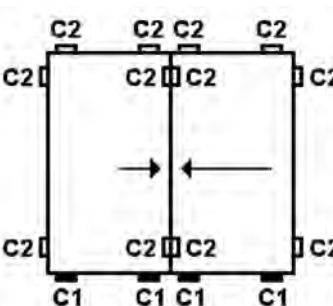
Figura 36. Cerco deslizante horizontal (corredera)
