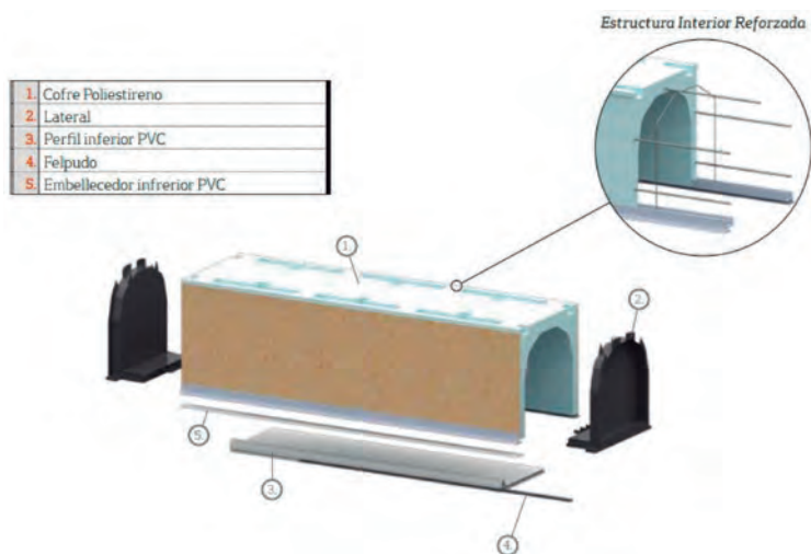
Figura 74. Partes del cajón túnel
