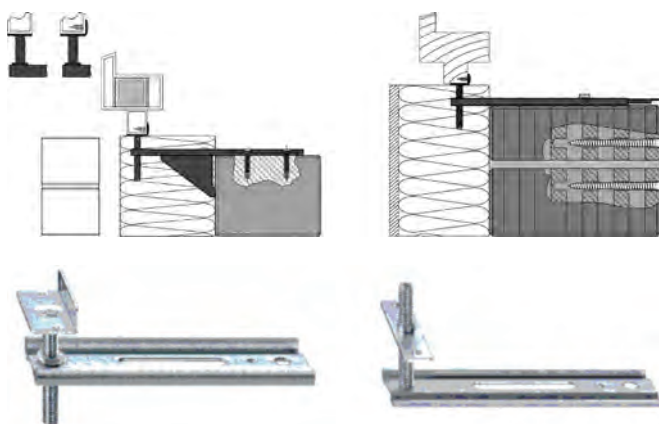
Figura 21. Consolas
