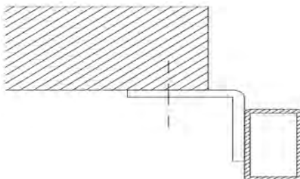
Figura 12. Anclaje sobrepuesto
