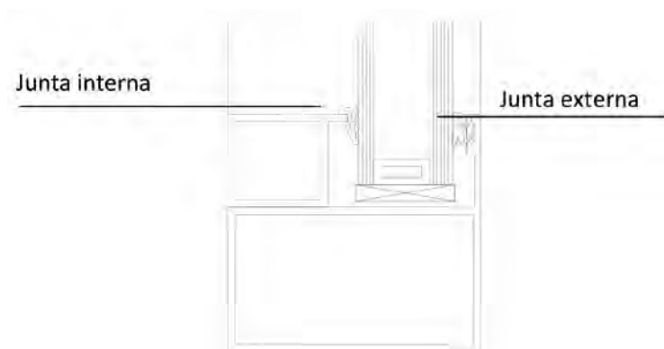
Figura 42. Junta interna y junta externa de acristalado
