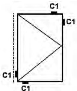
Figura 31. Marco practicable (Ventana abatible de giro vertical)
