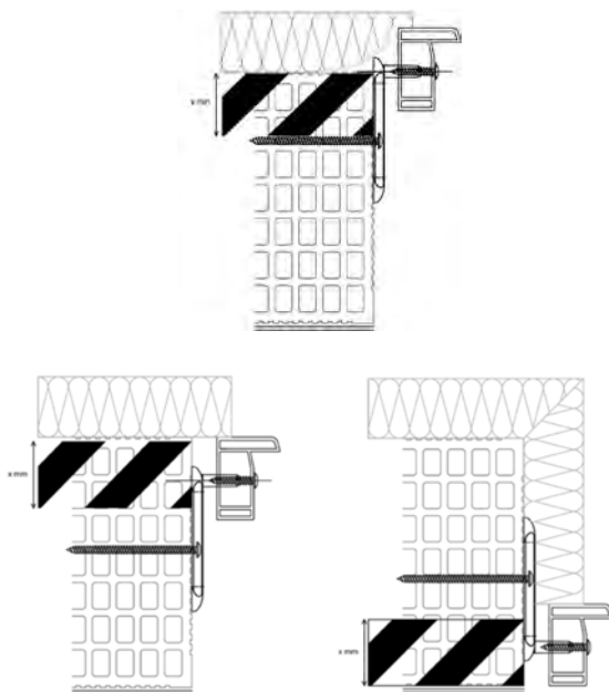
Figura 20. Fijación desplazada
